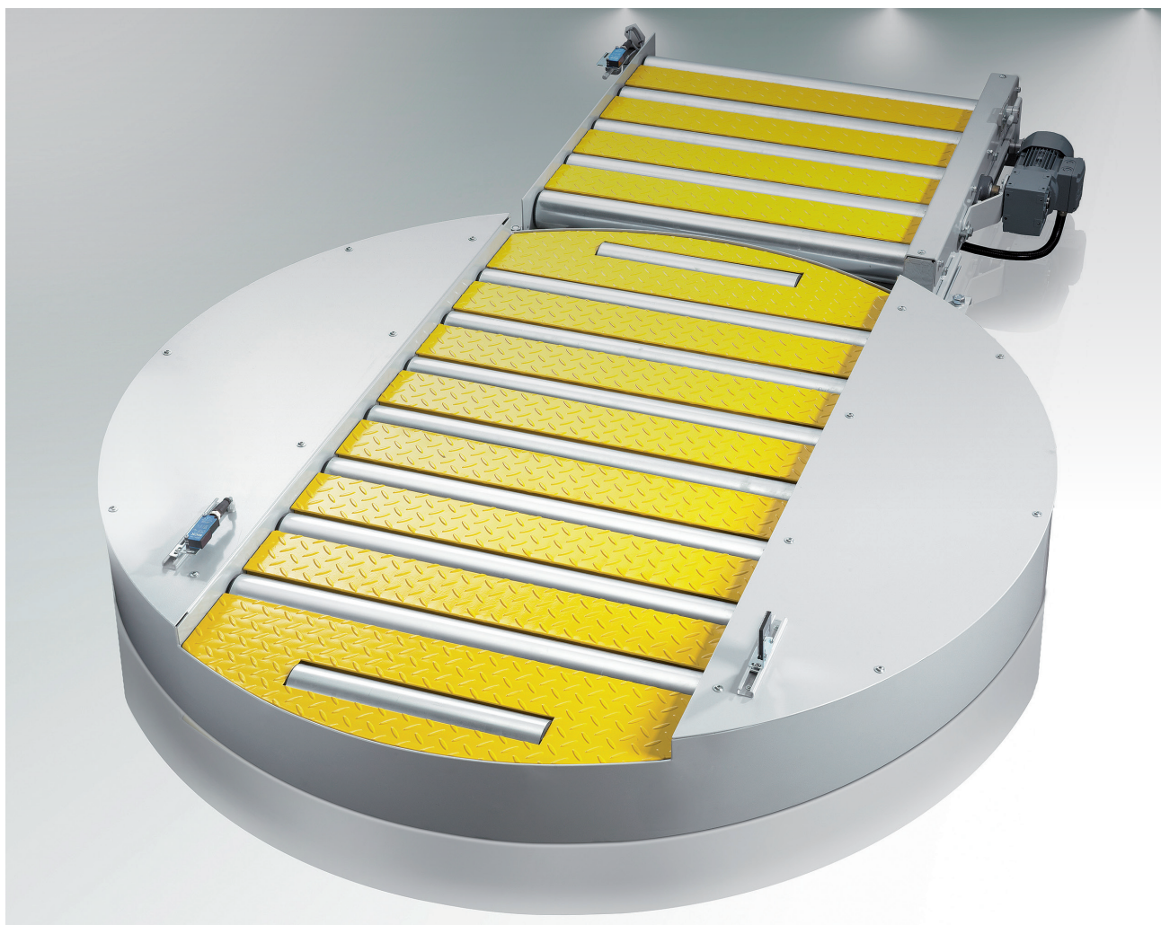
Kombination aus Trittblech für Rollenzwischenräume bei angetriebenen Rollenförderern ARF 80 / ARF 89 und Kompletteinhausung eines Drehtisches mit angetriebenem Rollenförderer DRF 80 / 89, welcher somit auch begehbar ist
