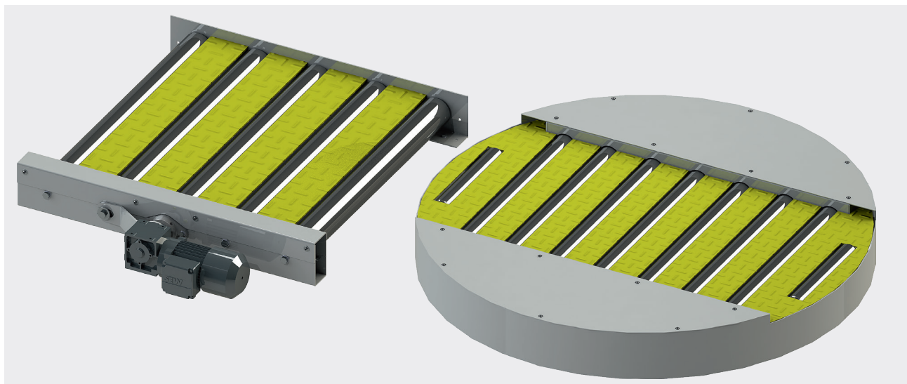
Trittbleche für Rollenzwischenräume bei angetriebenen Rollenförderern ARF 80 / ARF 89
